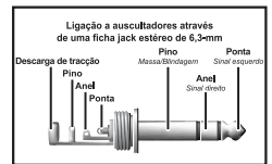
Fig. 5.4: Ficha jack estereó para auscultadores
