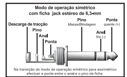
Fig. 5.3: Ficha jack estereó de 6,3-mm
